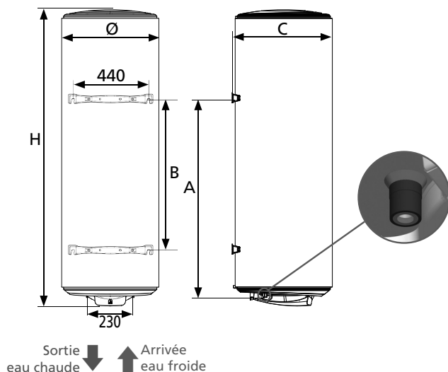
Représentation schématique
