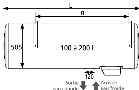
Représentation schématique
